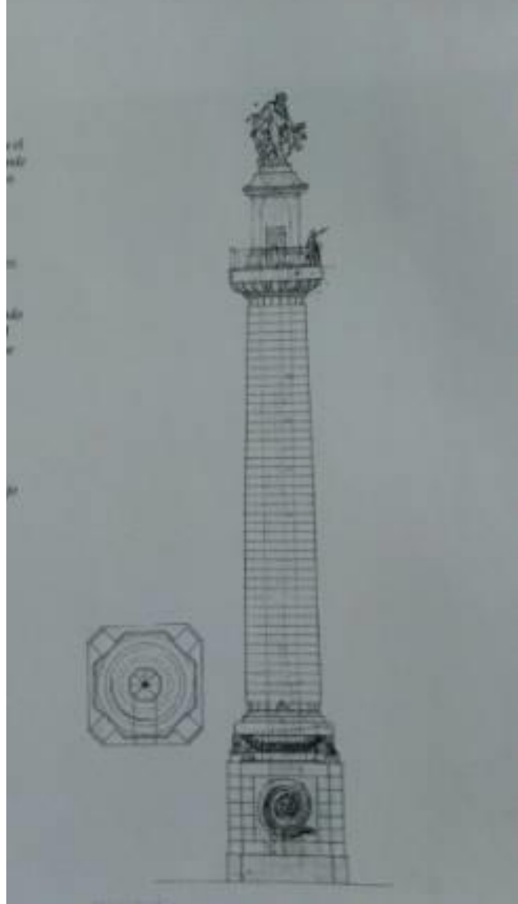
COLUMNA PROYECTADA, PERO NO REALIZADA, PARA EL CENTRO DEL ESTANQUE GRANDE DIBUJO DE ISIDRO GONZÁLEZ VELÁZQUEZ (AGP. PLANO 540)
