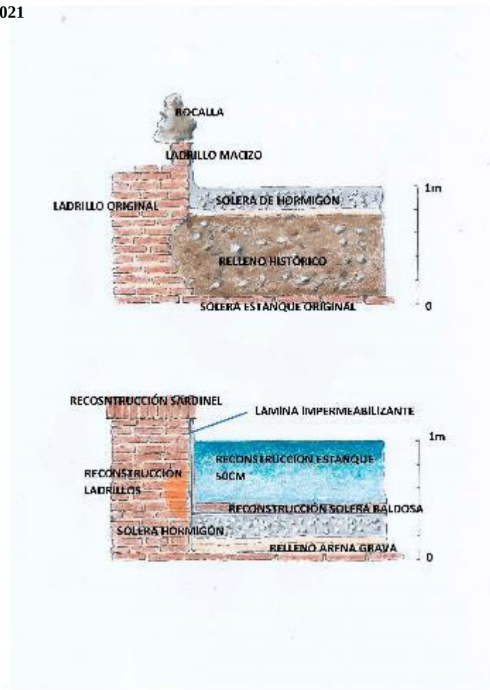
Arriba sección del estanque tras la excavación. Abajo, propuesta de consolidación del original y reproducción a una cota más elevada para respetar la profundidad de agua de 50cm
