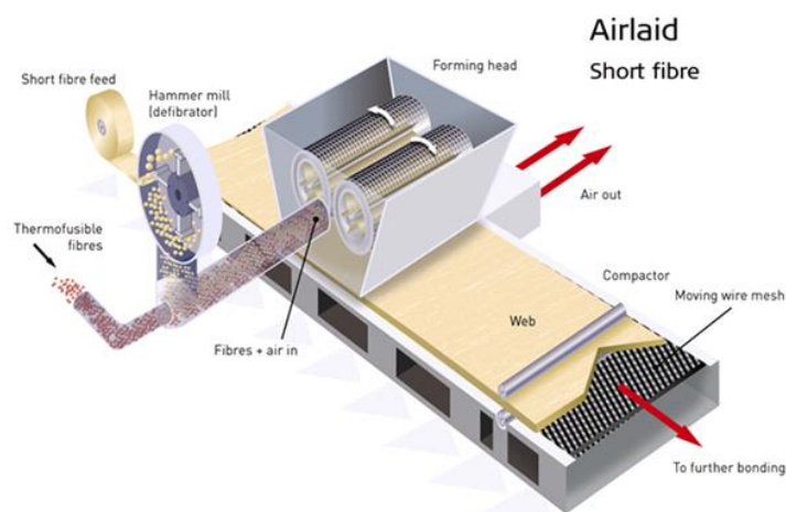
Imagen 9. Tecnología Airlaid
