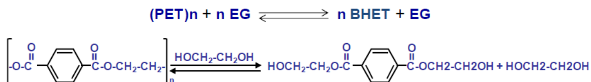
Imagen 3. Reacción química de glicólisis de poliéster
