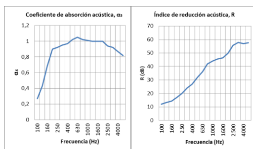
Figura 9 Ejemplo de curvas de absorción e índice de reducción acústica del material empleado
