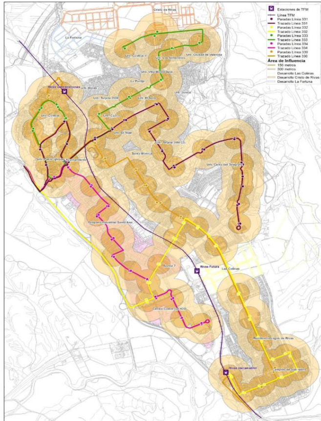
Ilustración 23 Cobertura de la red de transporte público interurbano según ordenación propuesta
