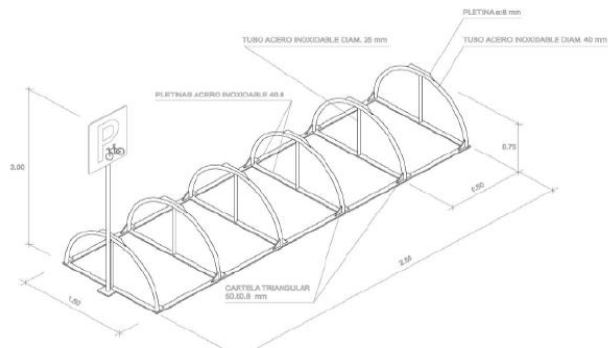
Ilustración 23 Modelo de Aparcamiento para Bicicletas
